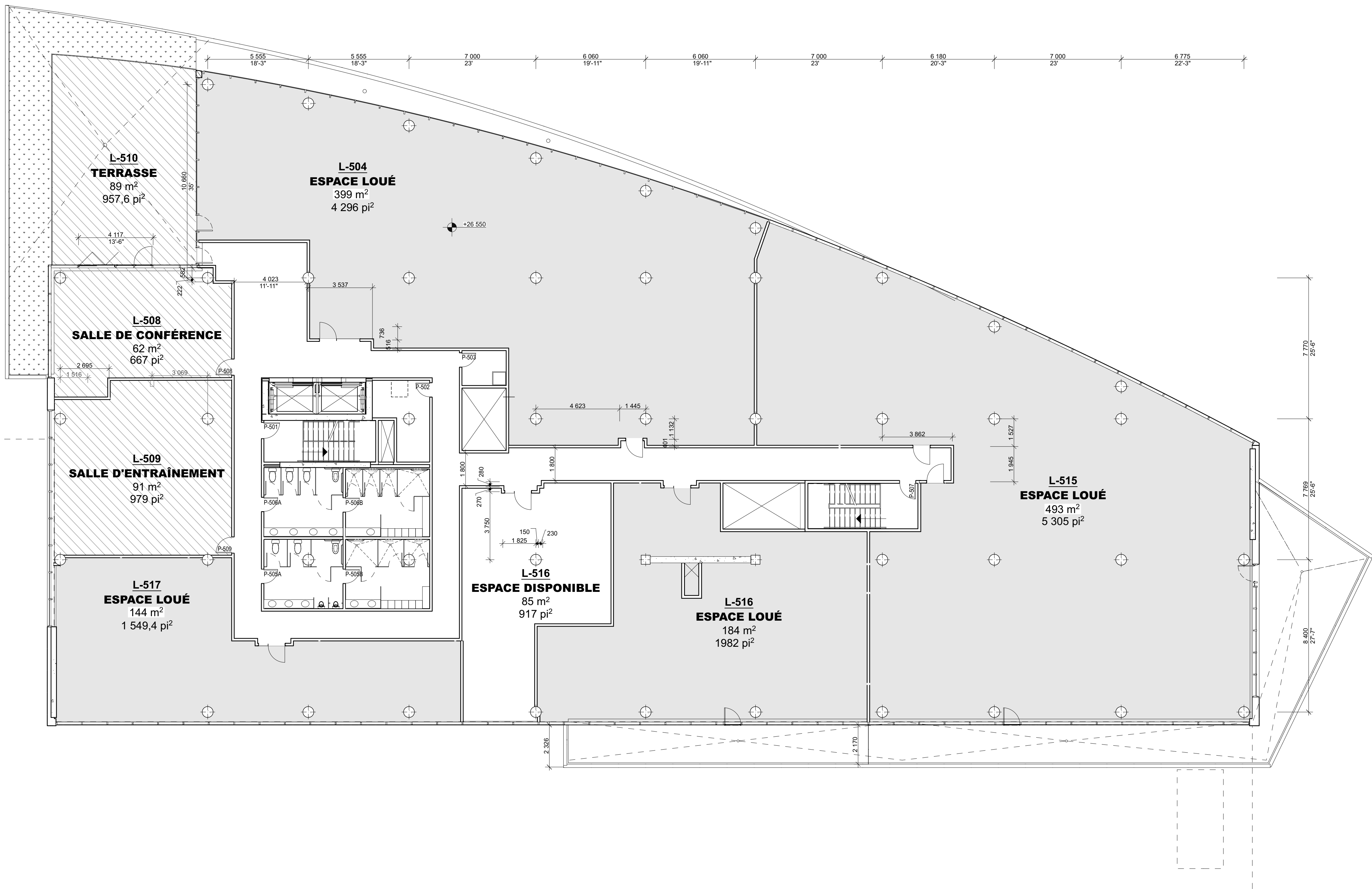
NIVEAU 5_PRÉSENTATION
